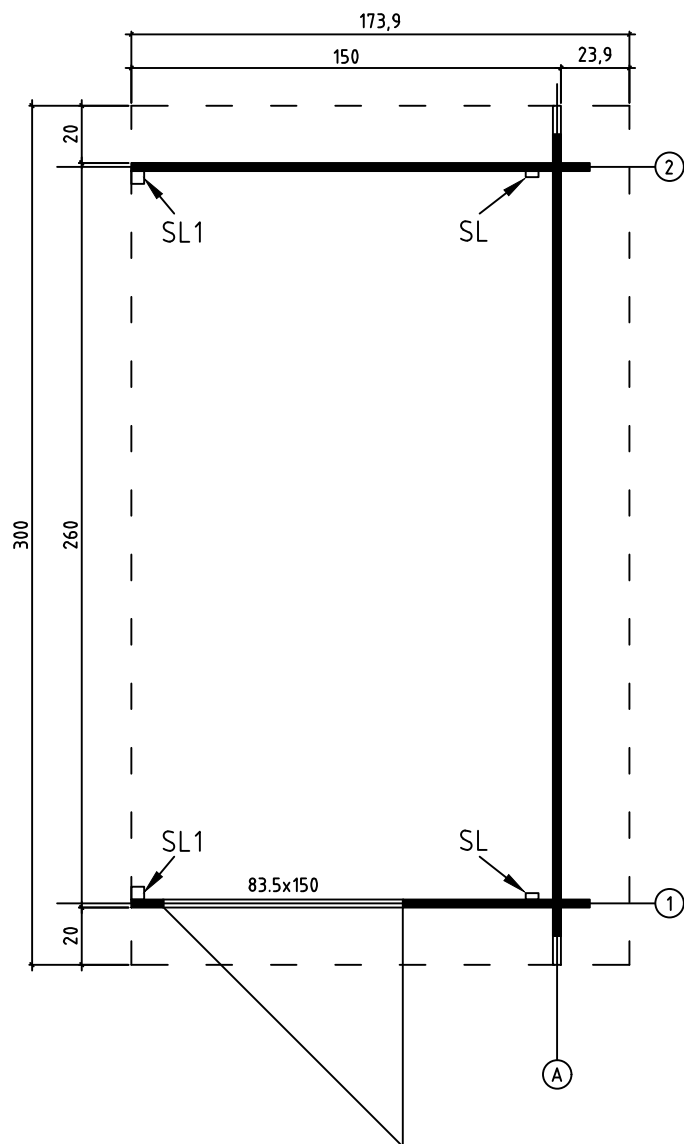
GROUNDPLAN - GRUNDPLAN - PLAN DE MASSE
